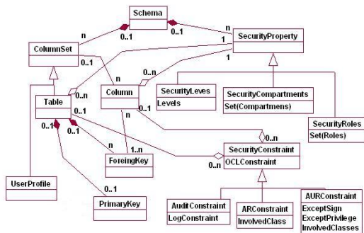
Figura 3. Metamodelo SECDW usado para diseñar el SMD PSM
