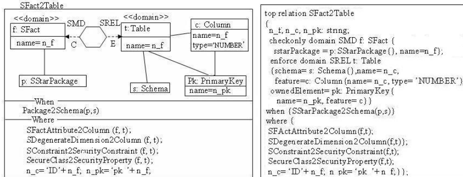
Figura 5. Transformando SFact en Table
