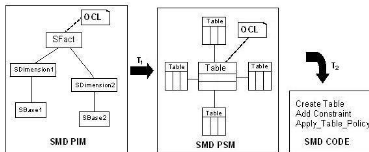
Figura 1. Obteniendo el SMD PSM y el SMD Code a partir del SMD PIM
