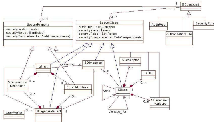
Figura 2. Metamodelo SECDW usado para diseñar el SMD PIM
