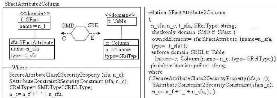
Figura 6. Transformando SFactAttribute en Column
