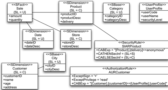
Fig. 8. PIM model.
